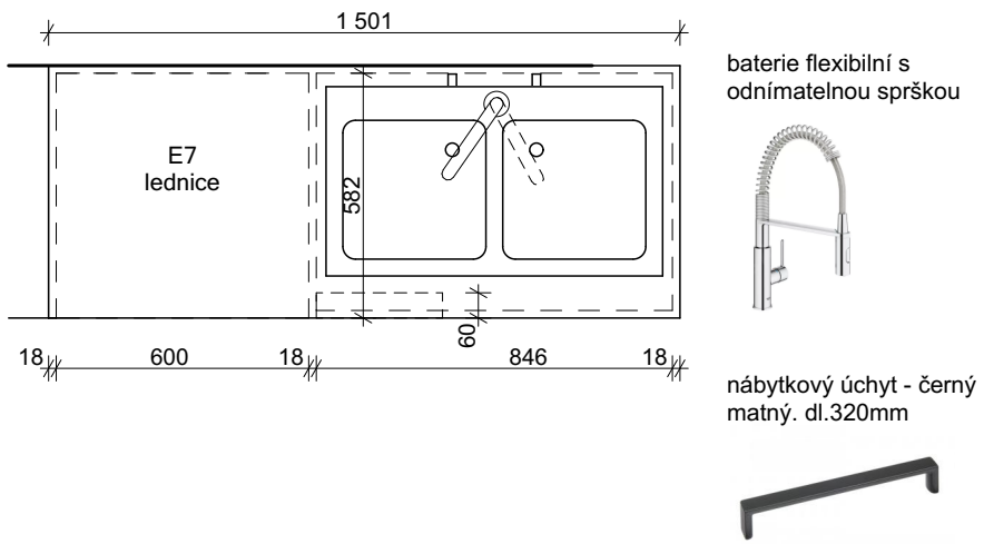
POHLED 1/20
