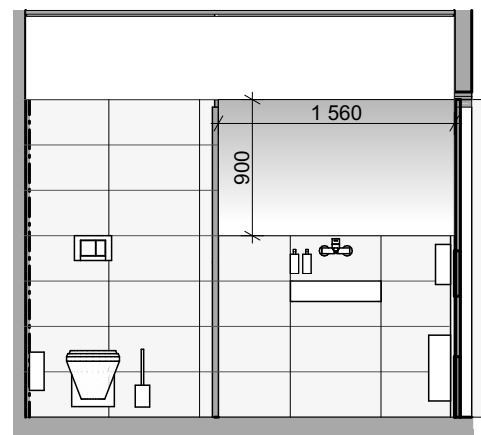
Pohled J1
