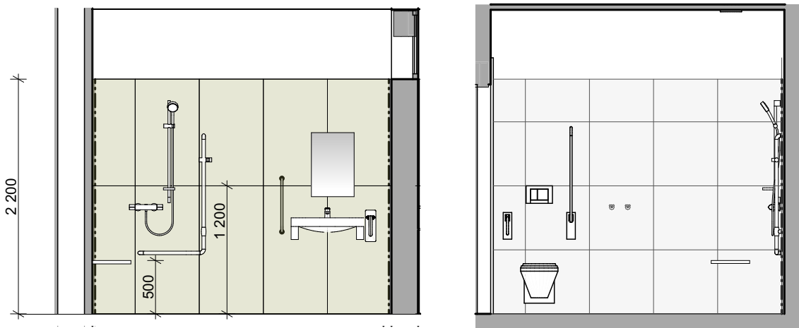
Pohled G1
