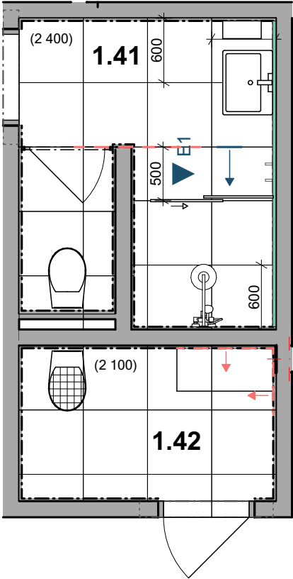
Půdorys - spárořez
