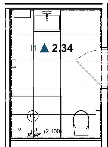
Půdorys - spárořez
