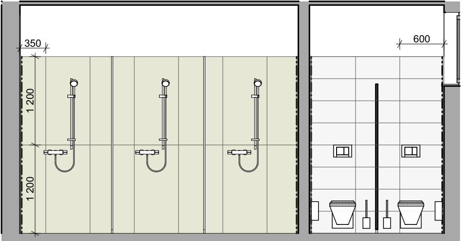
Pohled D1
