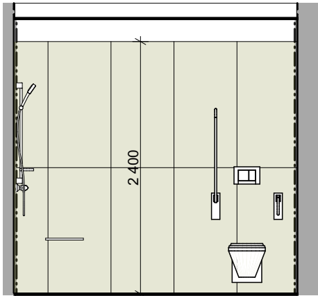
Pohled H1
