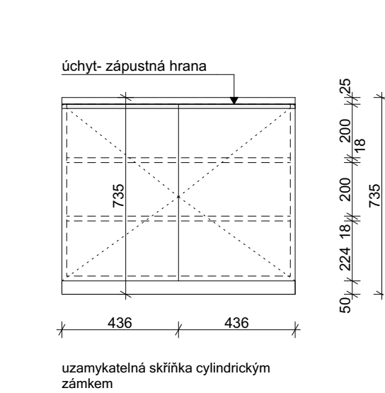
POHLED 1/20
