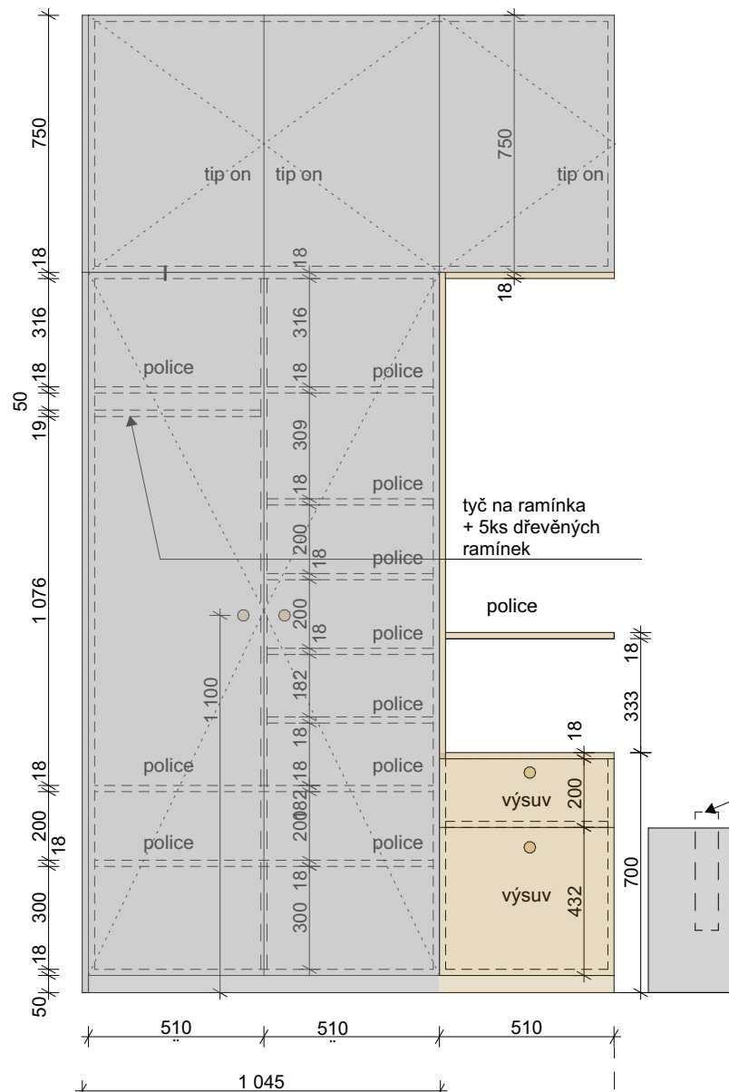
ROZVINUTÝ POHLED
