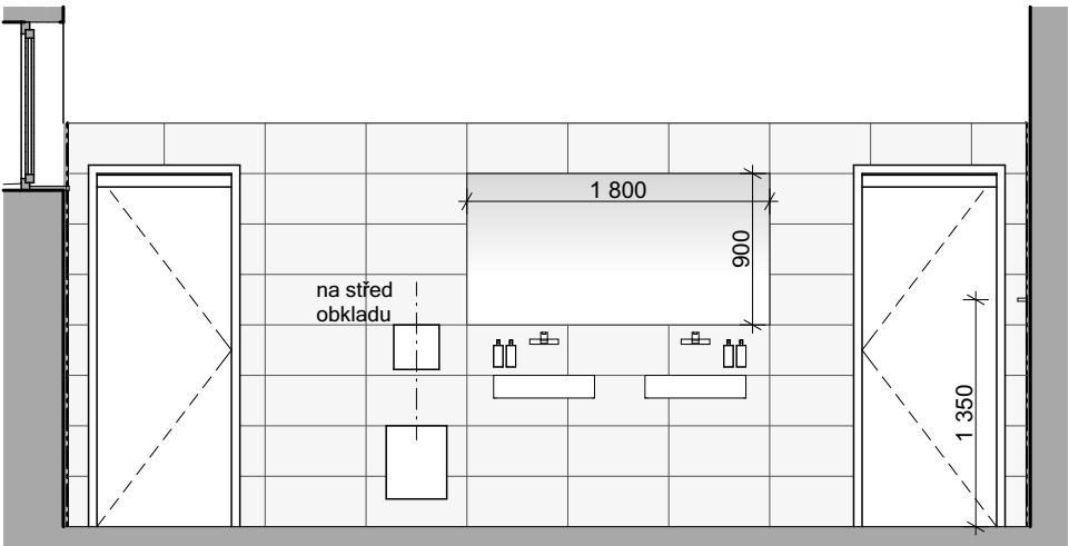
Pohled D2
