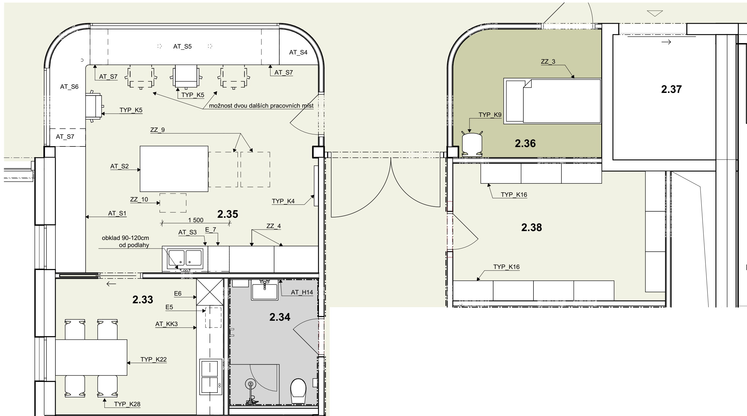
Půdorys - spárořez
