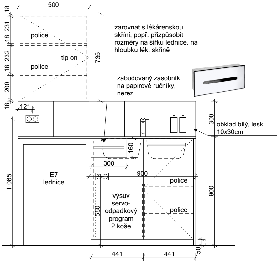
POHLED 1/20
