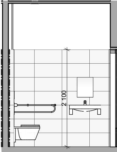
Pohled B3
