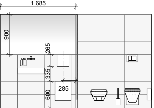
Pohled C2
