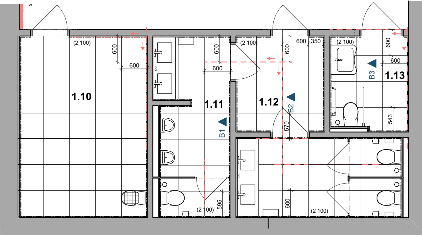
Půdorys - spárořez
