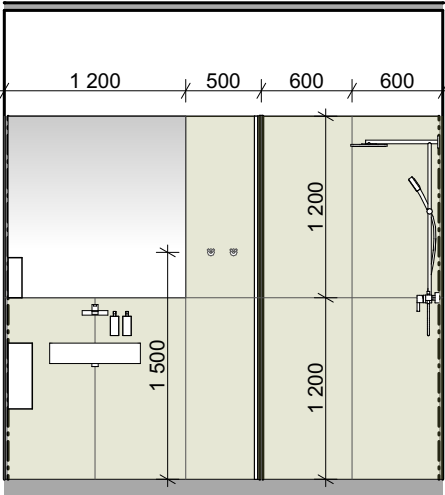
Pohled E1
