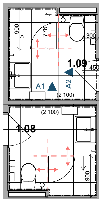
Půdorys - spárořez
