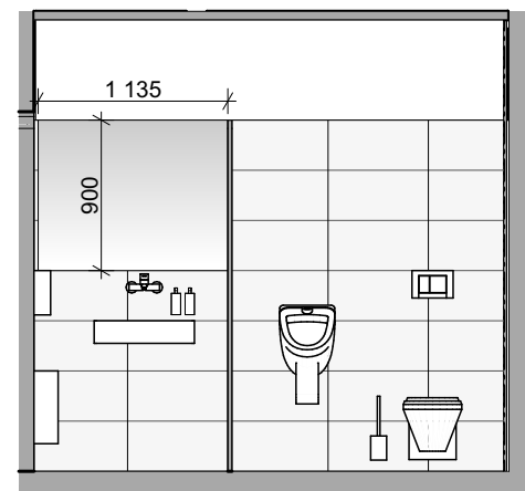
Pohled J2
