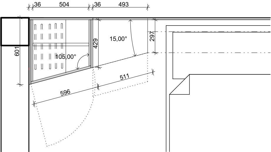
ROZVINUTÝ POHLED
