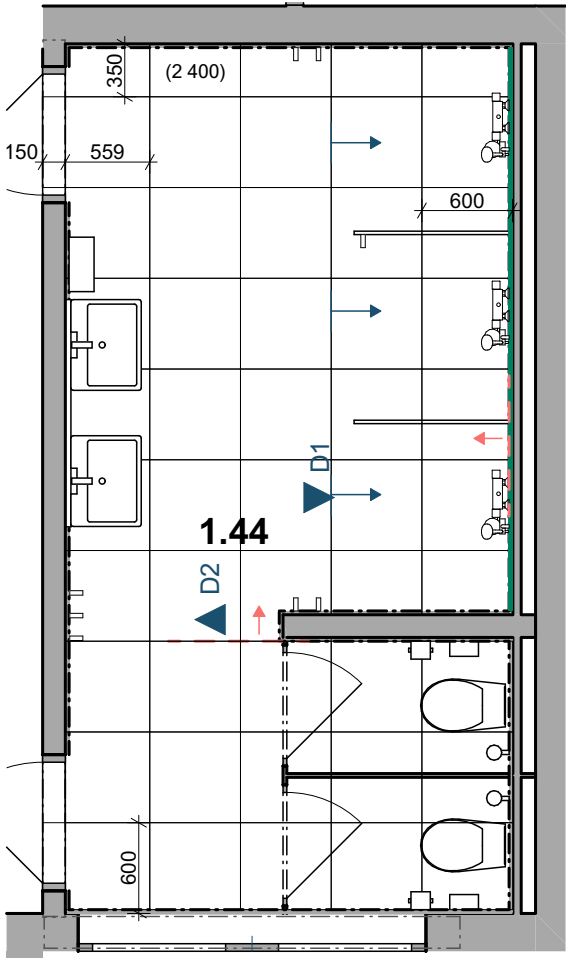
Půdorys - spárořez
