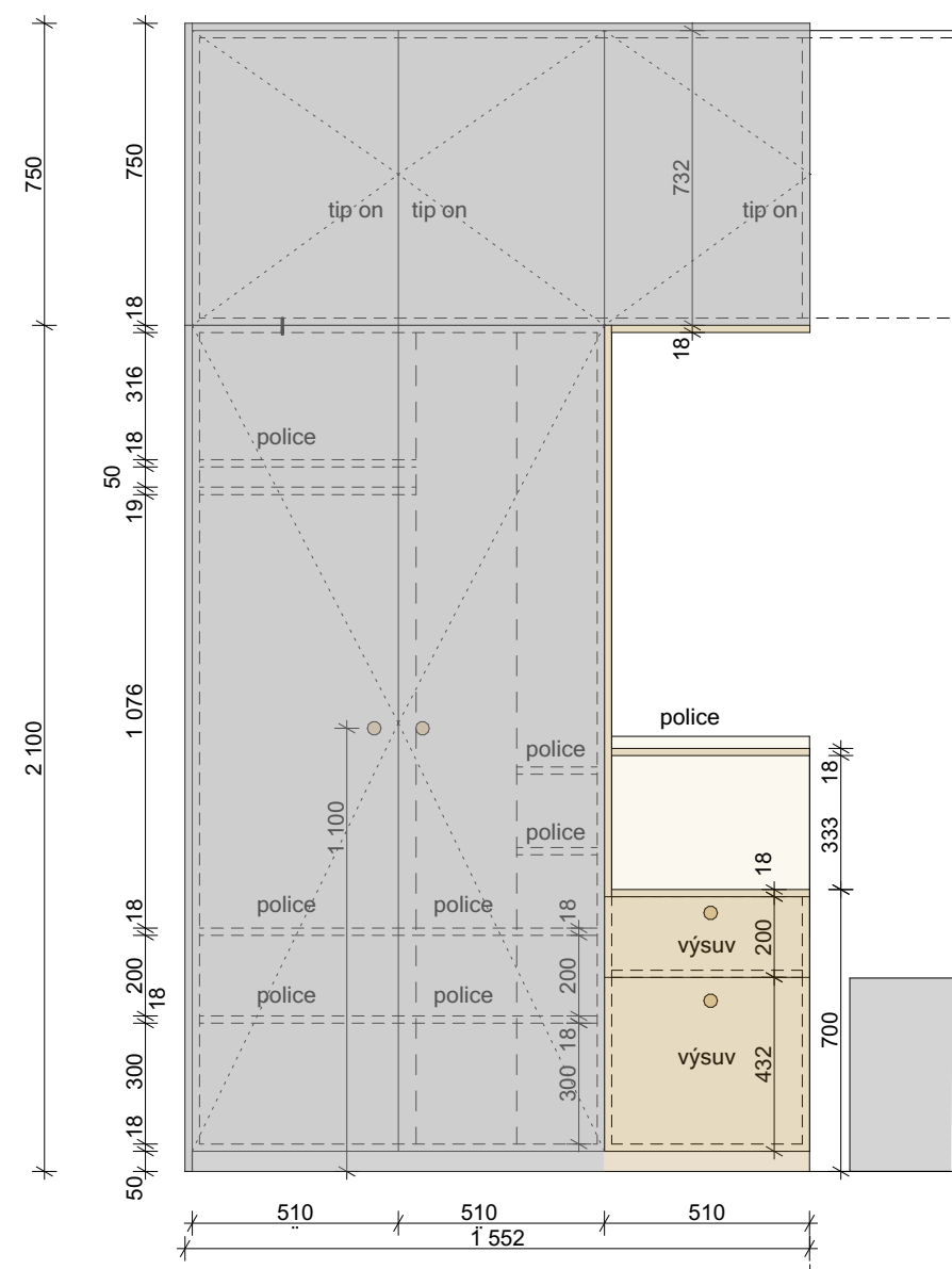
ROZVINUTÝ POHLED
