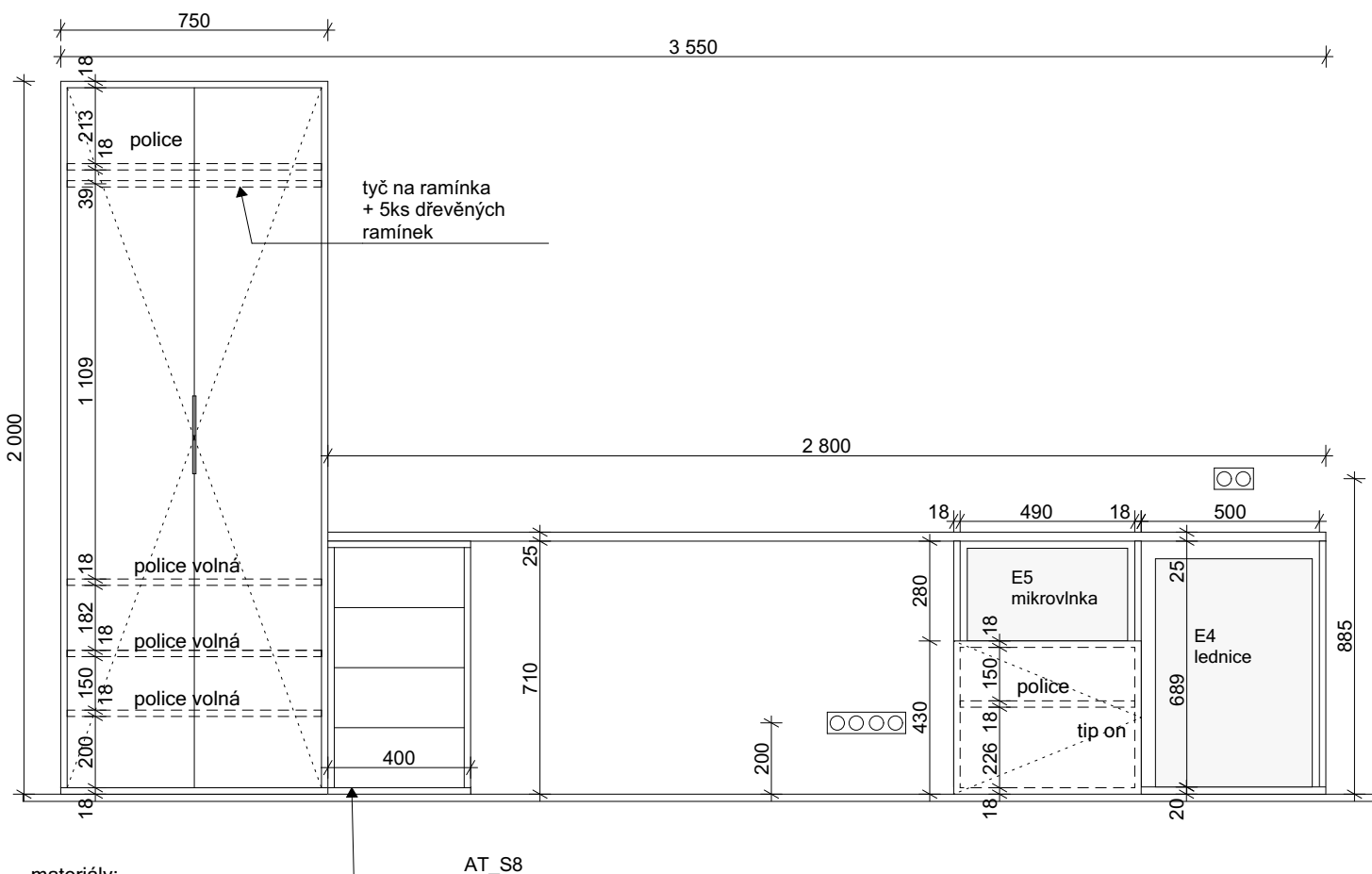
POHLED 1/20
