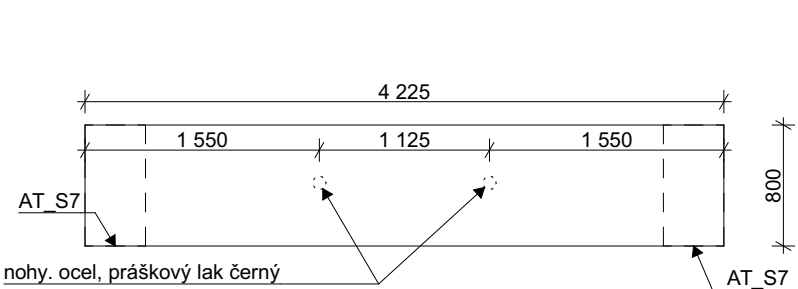
PŮDORYS 1/50
