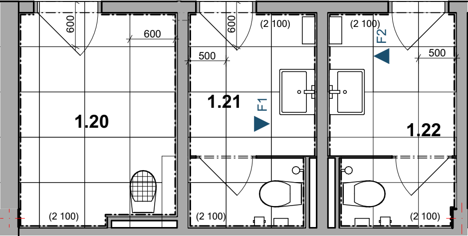
Půdorys - spárořez
