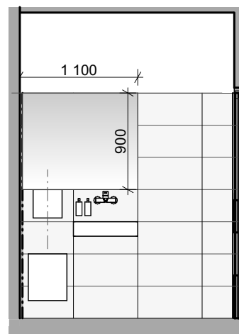
Pohled I1
