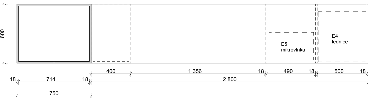
PŮDORYS 1/20
