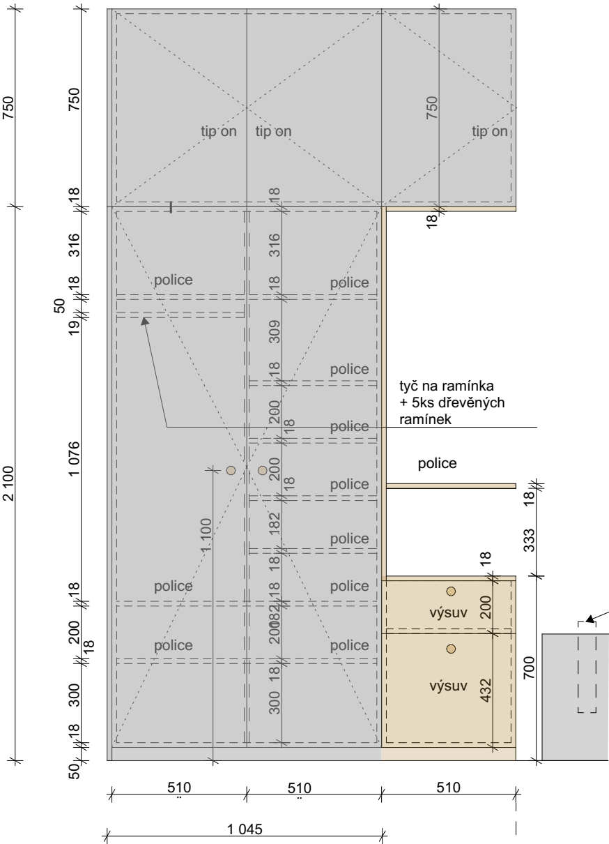
ROZVINUTÝ POHLED
