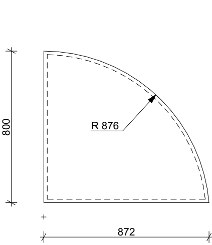
POHLED 1/20
