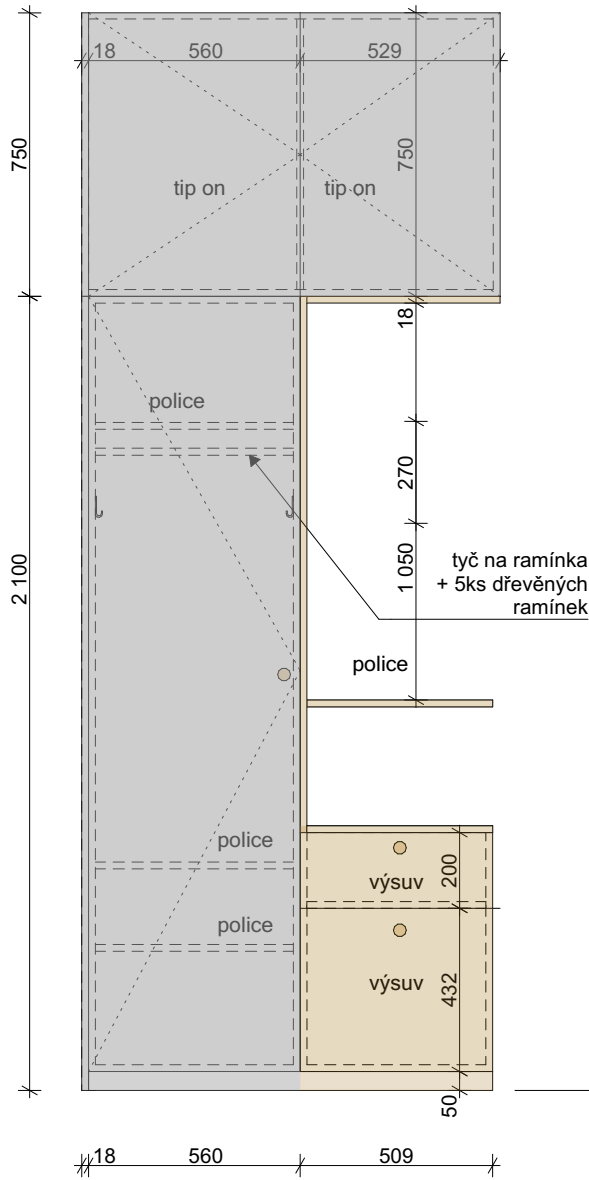
ROZVINUTÝ POHLED
