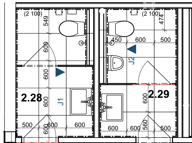
Půdorys - spárořez
