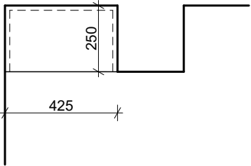
PŮDORYS 1/20 AT_K3
