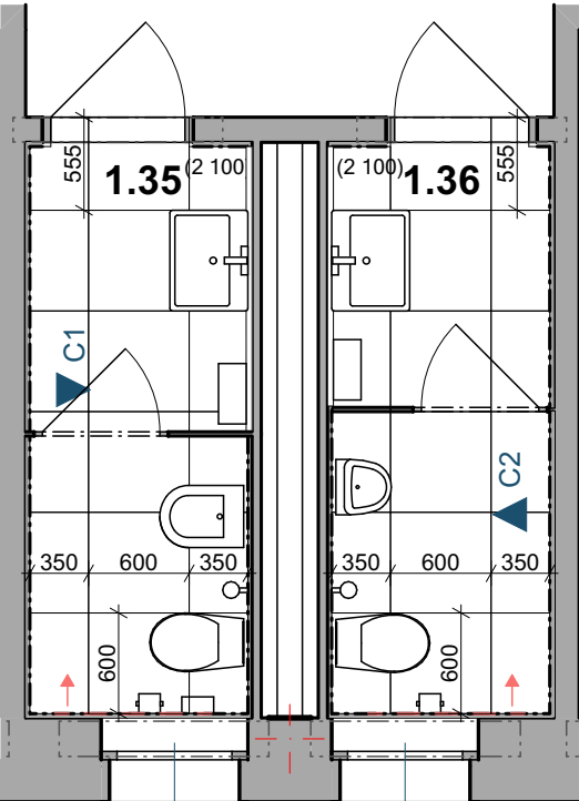
Půdorys - spárořez
