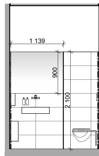
Pohled A2
