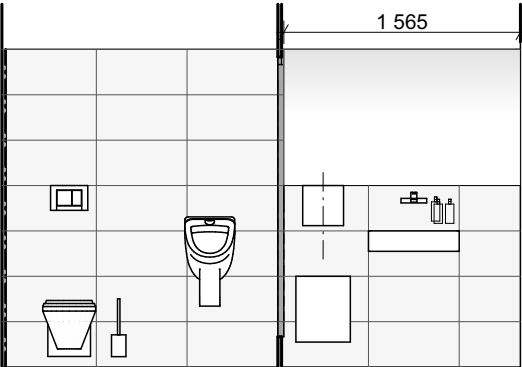
Pohled C1
