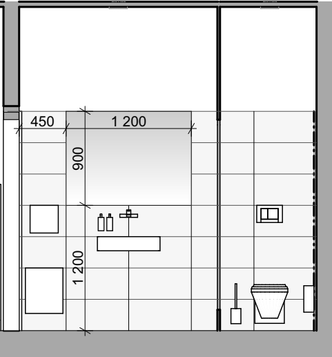
Pohled F1
