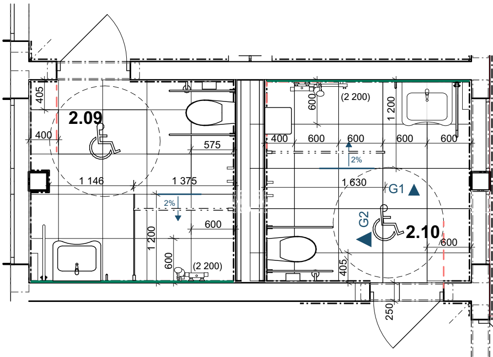
Půdorys - spárořez
